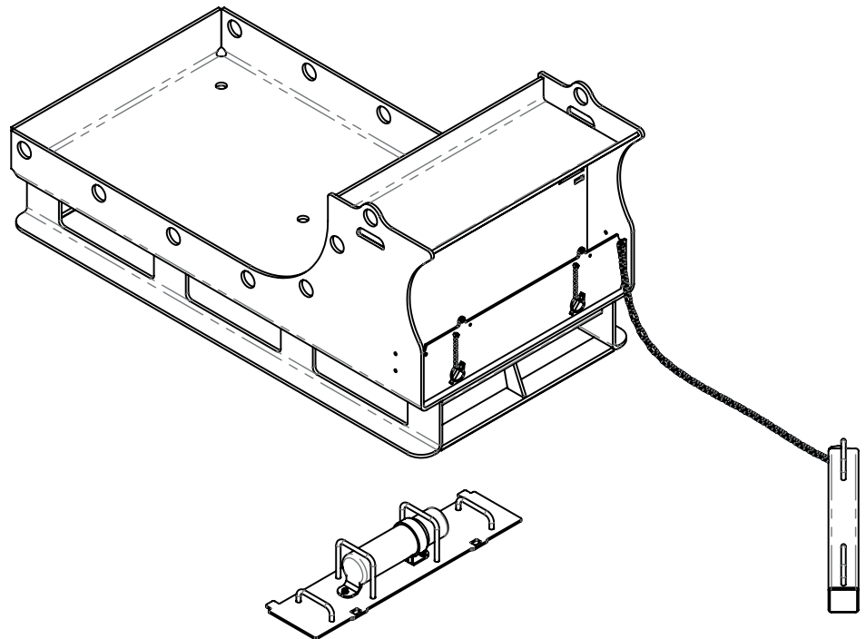
Transportgestell
