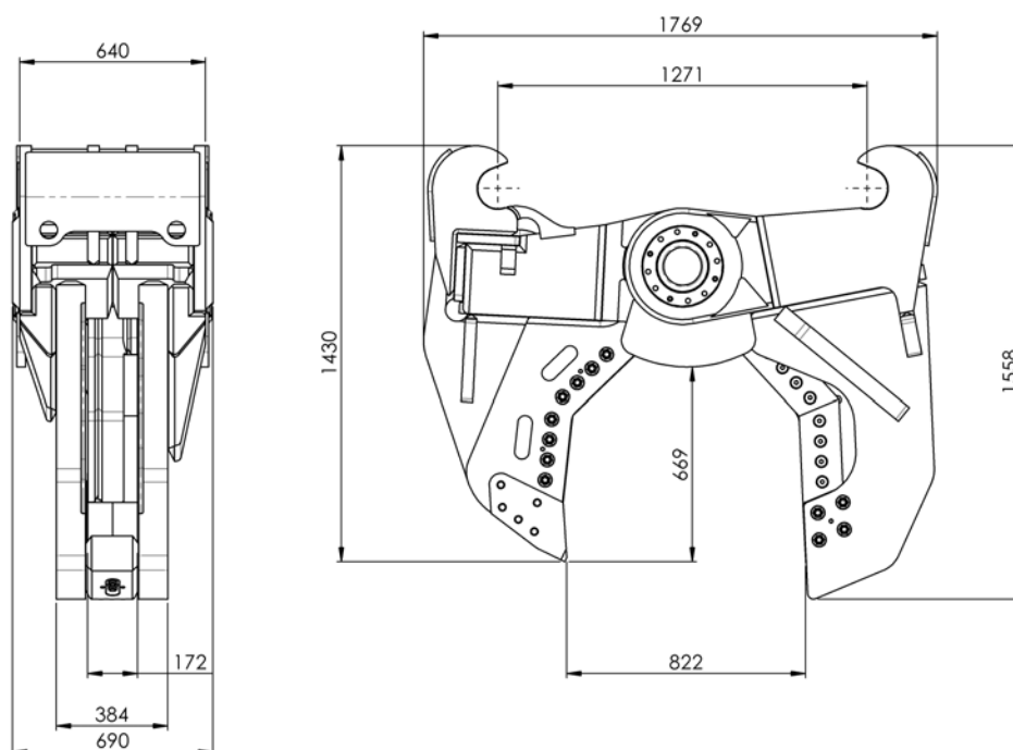
Stahl-Gebiss mit Doppelschneide
